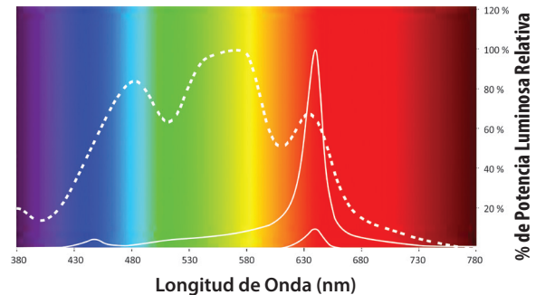
Salida Espectral de TLL Tubo Corto a 100% vs. 20%
