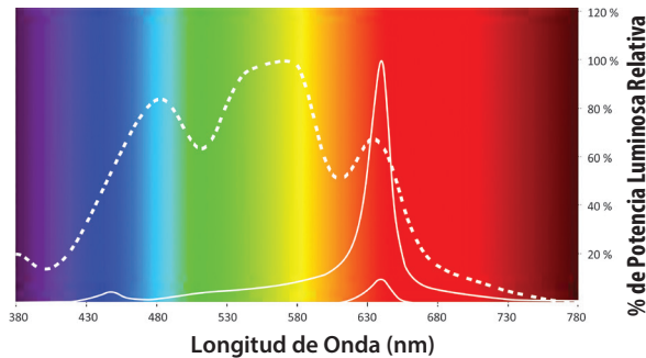
Salida Espectral de TLL Tubo Largo al 100% vs. 20%
